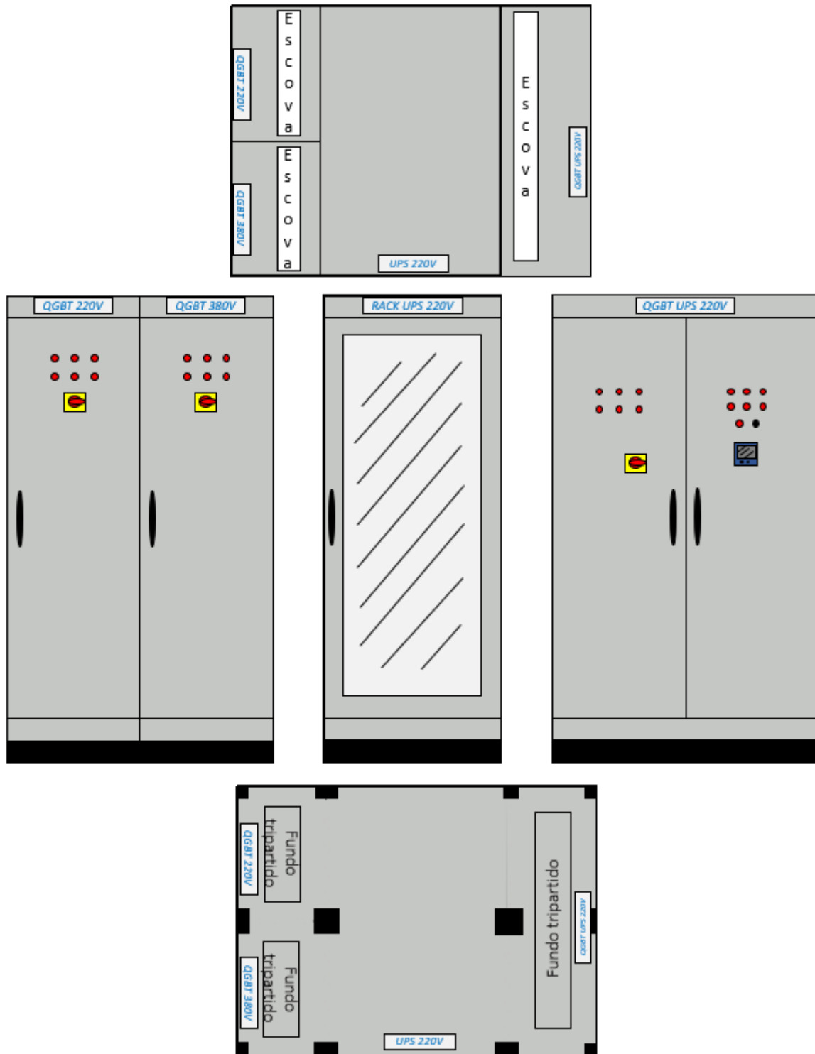
Figura 5 - Conjunto de painéis QGBT (ESB)
