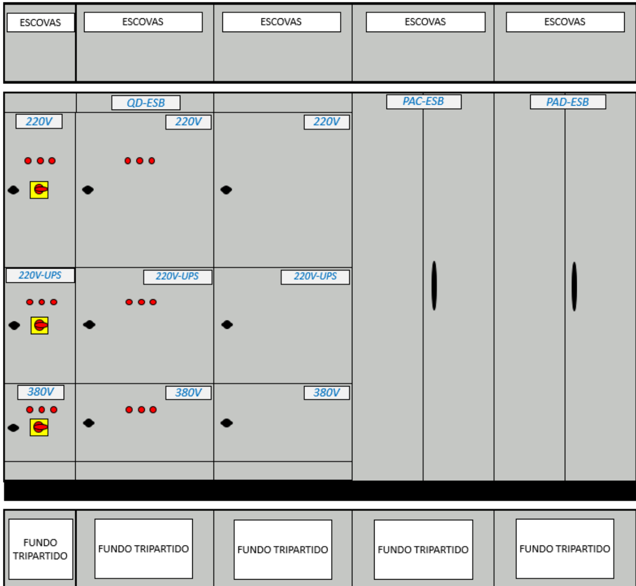
Figura 2 - Conjunto de painéis ESB
