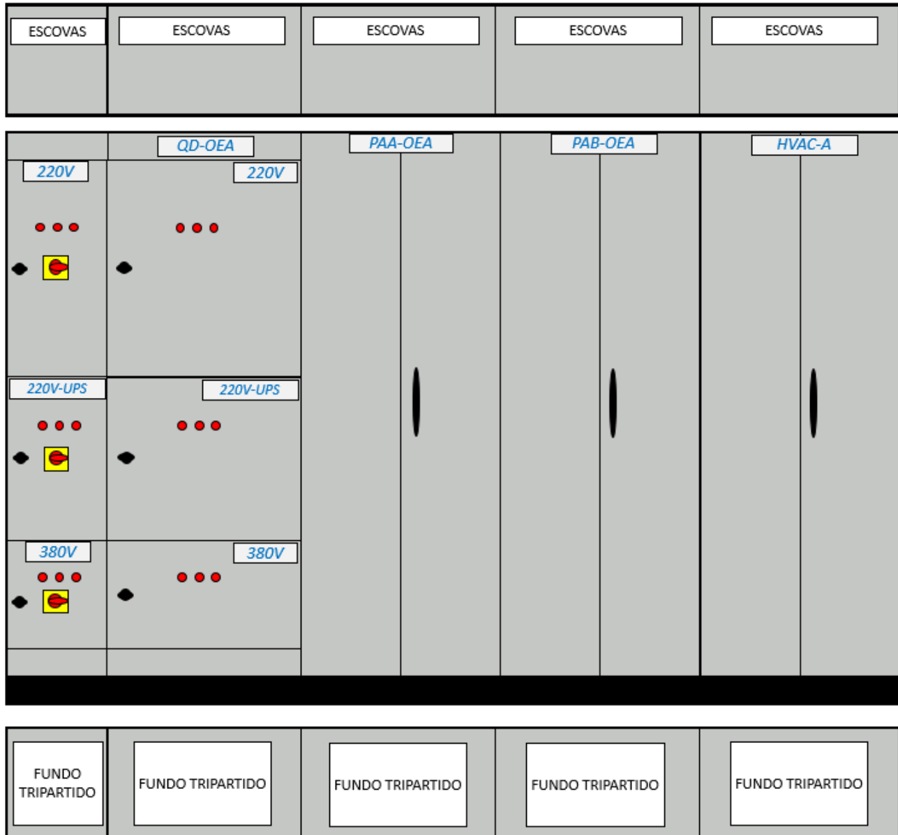
Figura 1 - Conjunto de painéis OEA
