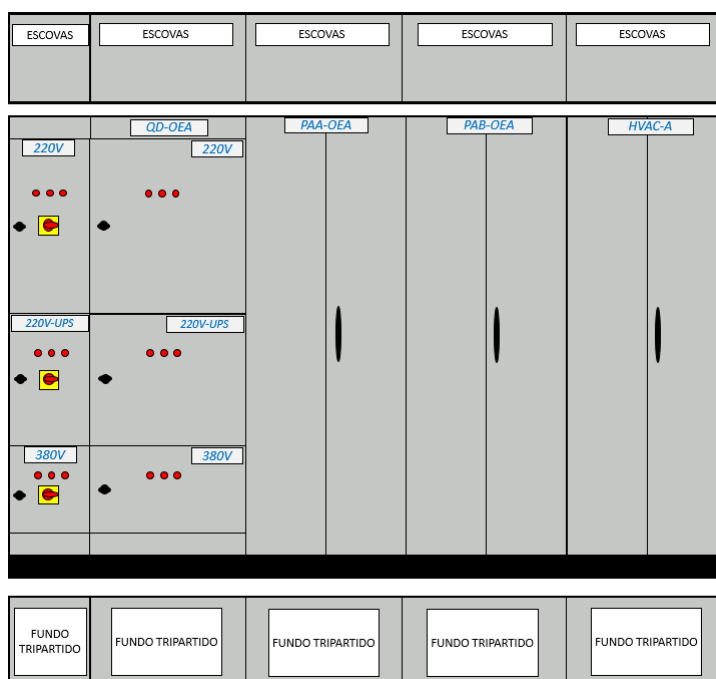
Figura 1 - Conjunto de painéis OEA
